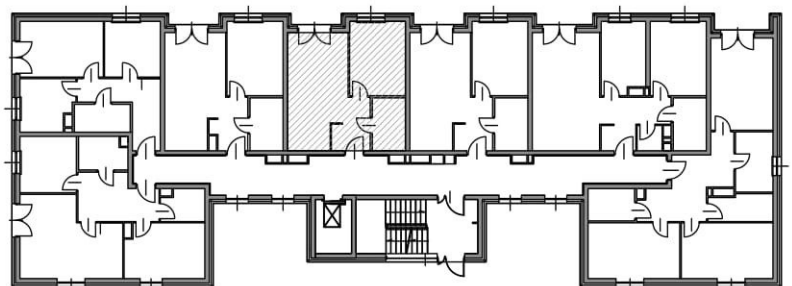
RZUT PARTERU
